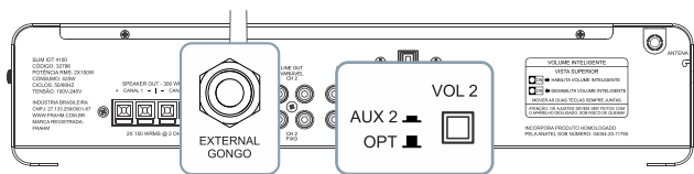
Conexão com plugue P10
